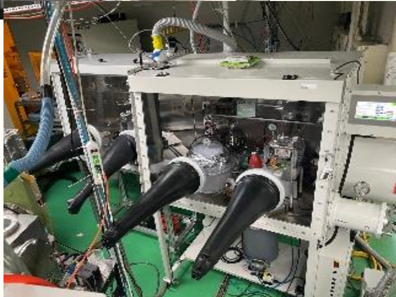
OLED蒸鍍系統 與 手套相連結
